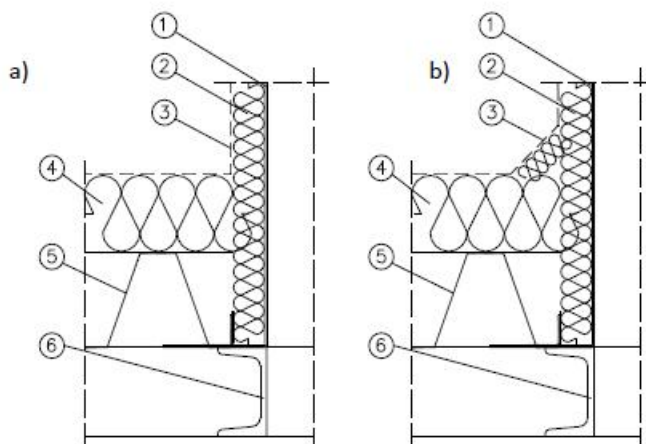
Рис. 7. Стальное основание на стальной конструкции (а – обработка мембраной, б – обработка рубероидом) 1 - стальное основание; 2 - термоизоляция основания; 3 - обработка мембраной или рубероидом; 4 - термоизоляция крыши; 5 - профилированные металлические листы; 6 - несущая стальная конструкция
